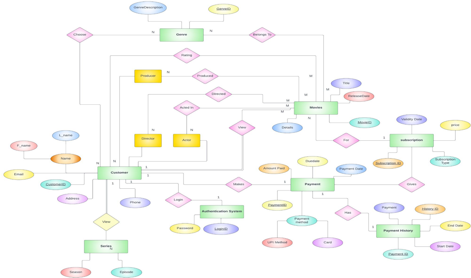
ER Diagram
